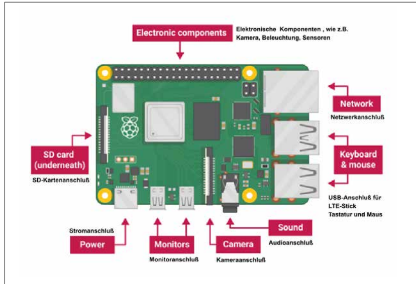
Raspberry Pi 4 Funktionsschaltbild (2020)
